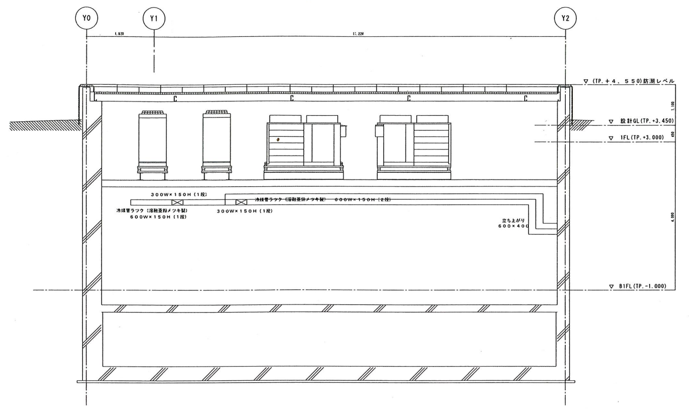
屋外機置場 A-A断面詳細図
