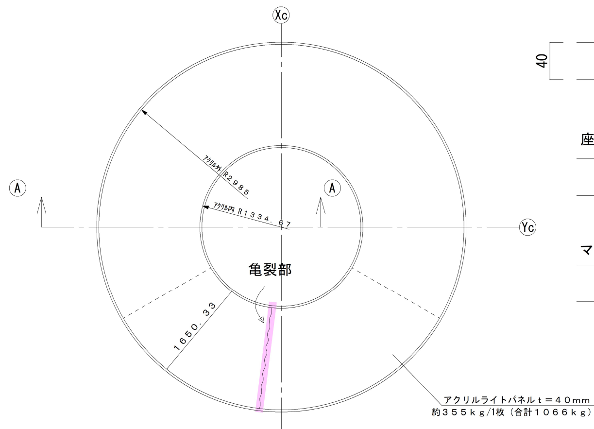
平面図 (S=1:60)
