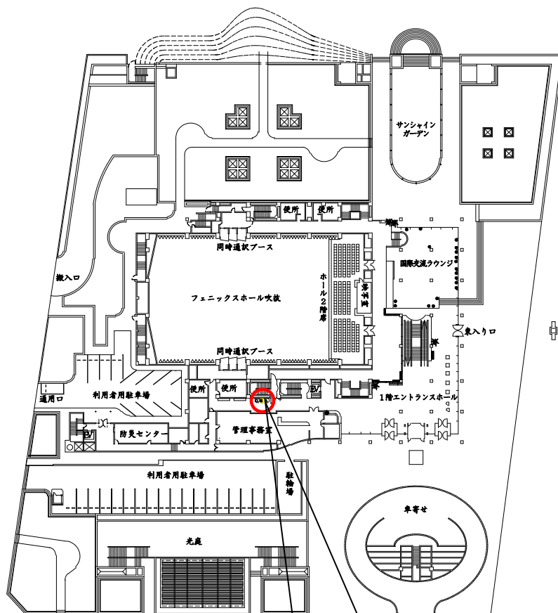
1 階平面図
