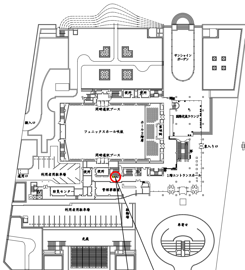
1 階平面図
